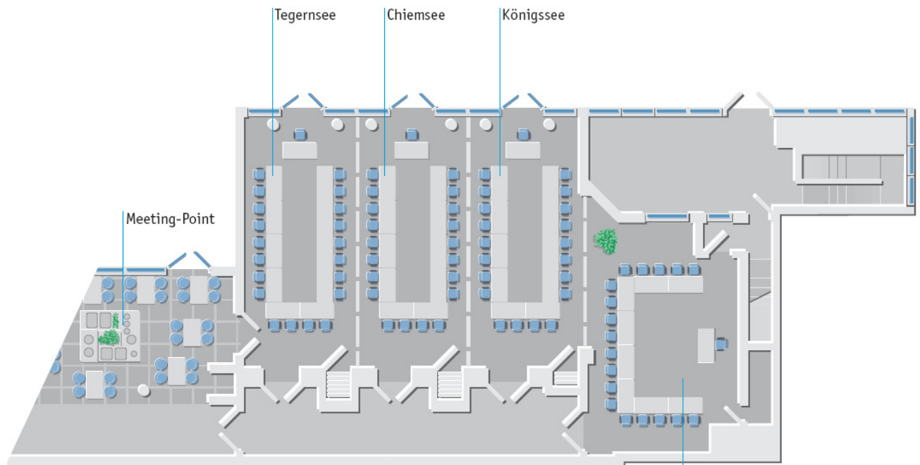
Konferenzzentrum, EG
